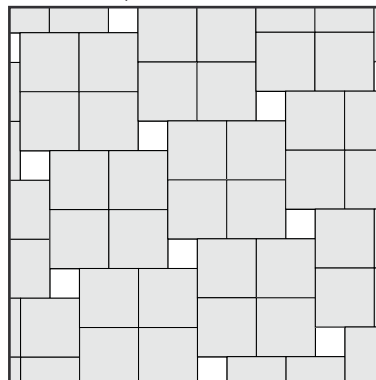
VZOR PDN 9 / DLAŽBA TAĀTĀNA
